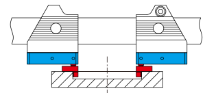
测量内径
