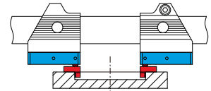
测量内径
