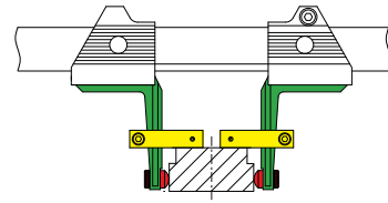
测量外径(球面测头)
