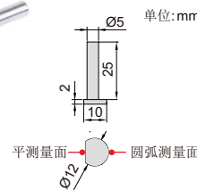
圆弧测量面测量孔内凹槽 直径(深度≤3.5mm)
