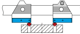
测量中心距
