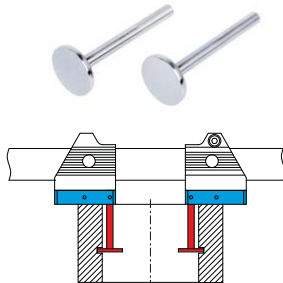
测量孔内凹槽直径(深度≤7.5mm)
