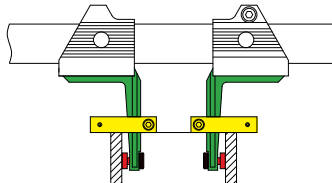
测量内尺寸(平测头)
