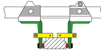
测量外尺寸(平测头)
