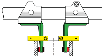
测量内径(球面测头)
