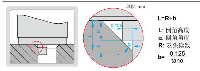
测量原理
