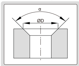
测量沉孔口端直径
