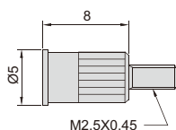
平测头
