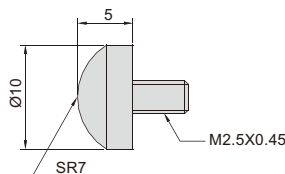
球面测头
