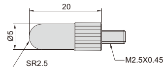
壳型测头
