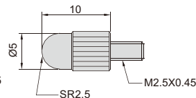
壳型测头
