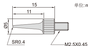
针测头
