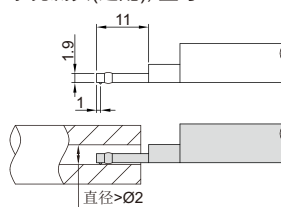
深沟槽测头(选配), 型号 ISR-C002-DGP
