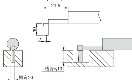
深沟槽测头(选配), 型号 ISR-C002-DGP
